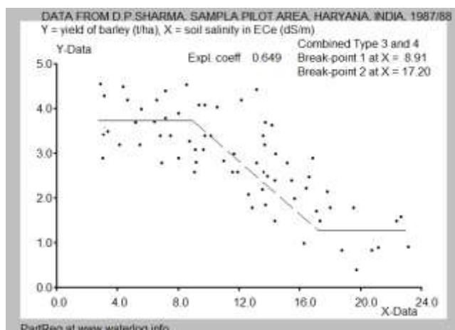
Fig. 3.1 Barley. BP=9 dS/m
