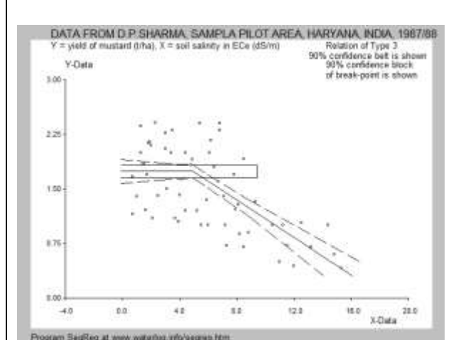
Fig 4.2 Mustard (rapeseed). BP=5 dS/m
