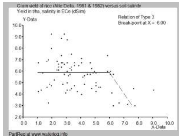
Fig. 1.4 Rice. BP=6 dS/m
