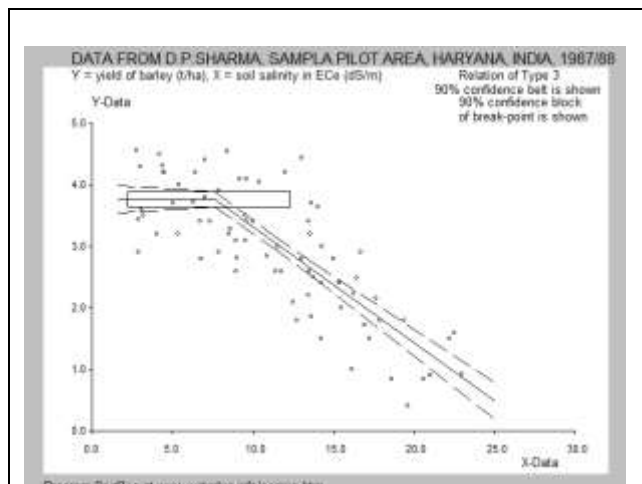
Fig. 4.1 Barley. BP=7.6 dS/m
