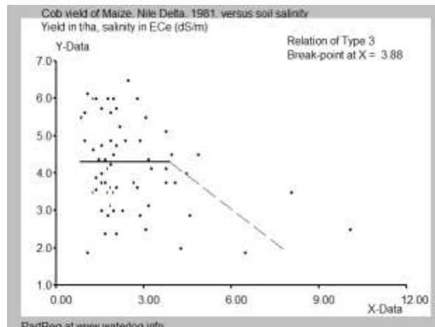
Fig. 1.3 Maize. BP= 4 dS/m
